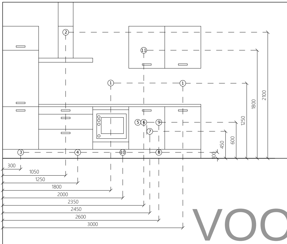
vooraanzicht
